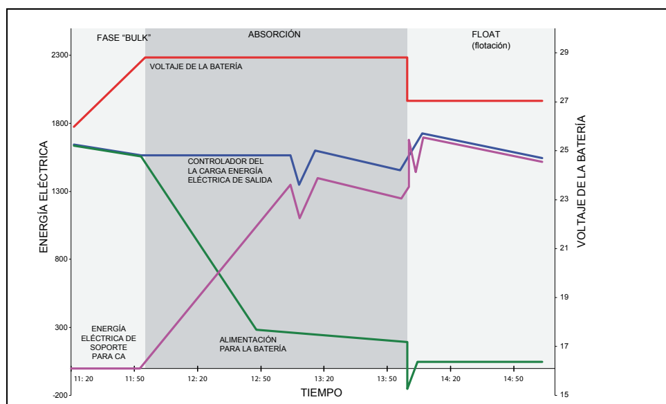
Figura 4 Ciclo de carga del Soporte de CA mejorado
