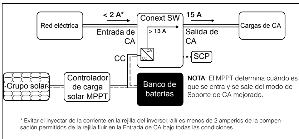
Figura 3 Soporte de CA mejorado
