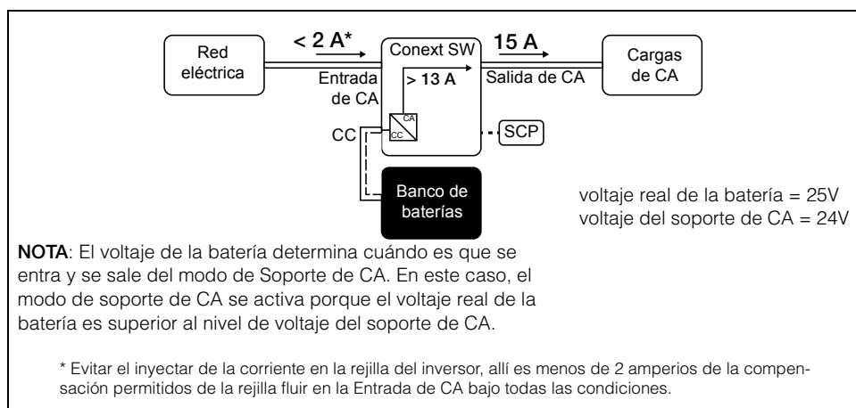
Figura 5 Soporte de CA normal sin dispositivos Xanbus
