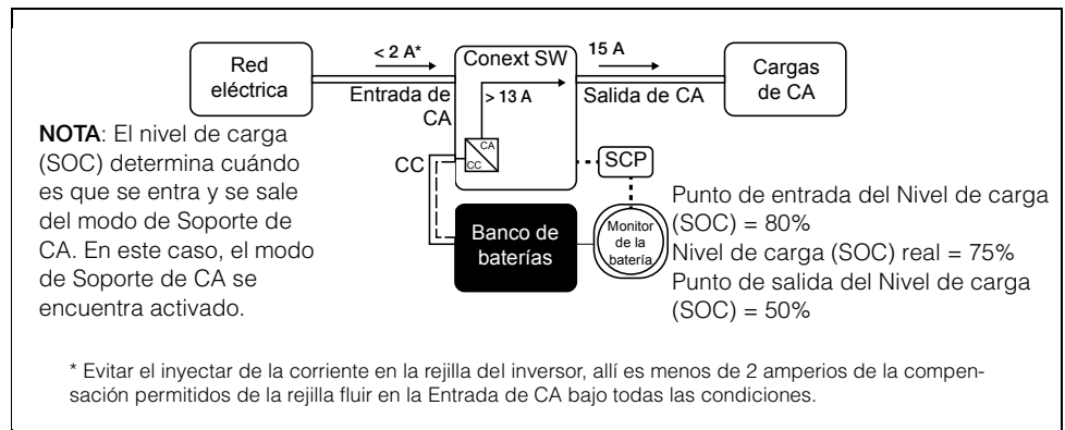
Figura 2 Modo de Soporte de CA utilizando Nivel de carga (SOC)
