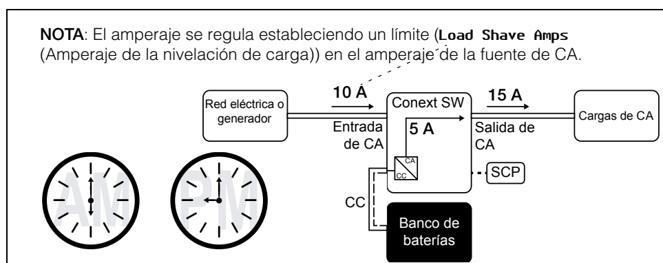
Figura 1 Nivelación de cargas en acción
