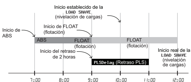
Figura 6 Ejemplo del retraso de 2 horas de la nivelación de cargas
