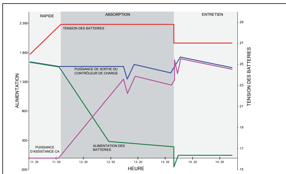
Figure 4 Cycle de charge avec assistance CA améliorée
